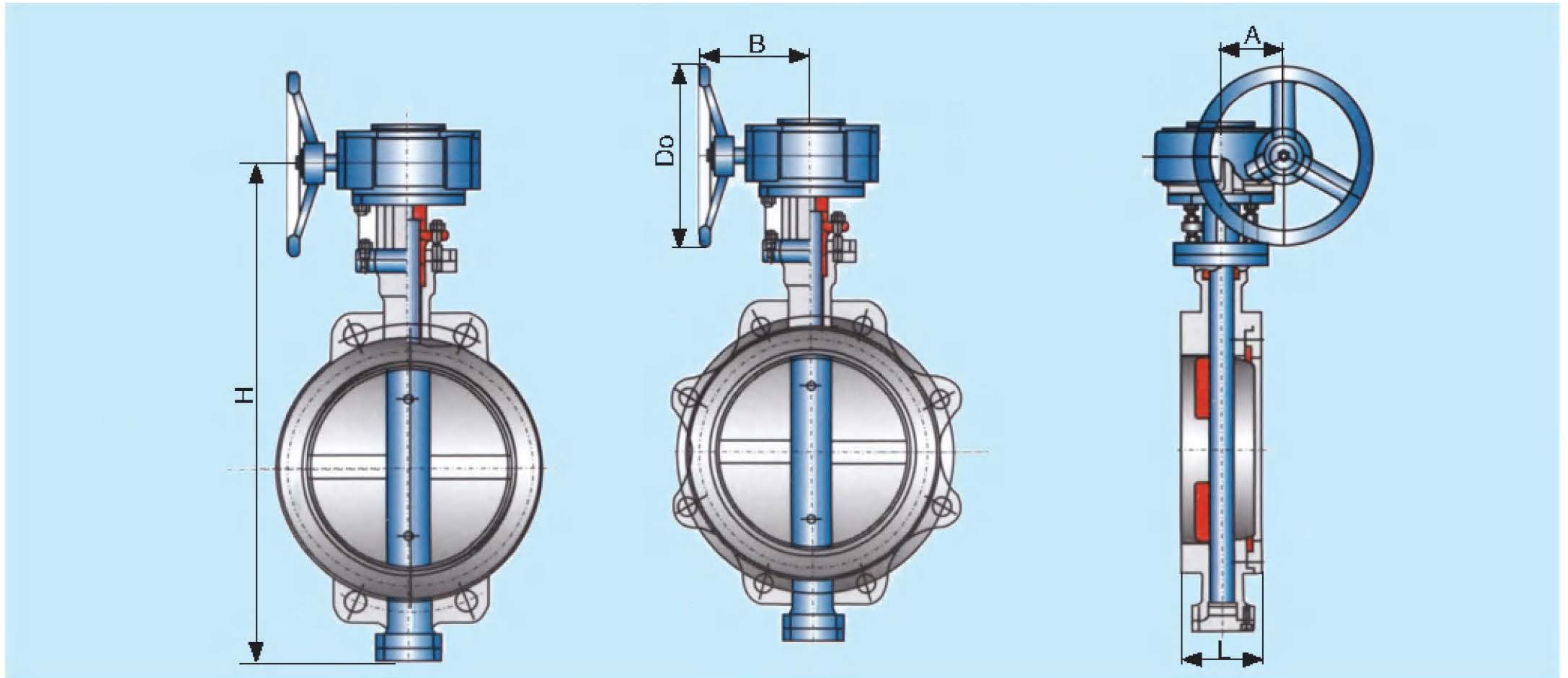
外形尺寸 Overall dimensions ( mm ) ANSI Class 150Lb
